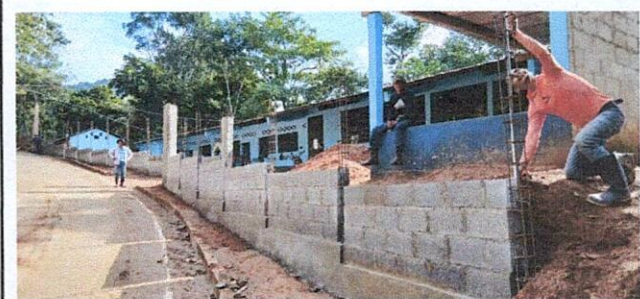
Foto 6: preparación de las columnas para su fundición
